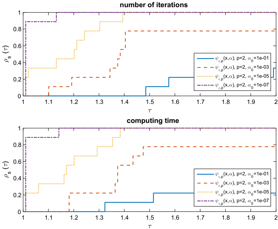
Fig. 5 Performance profile of \psi_{\varepsilon,p} when \alpha_0 = 1e - 1, 1e - 3, 1e - 5 and 1e - 7
