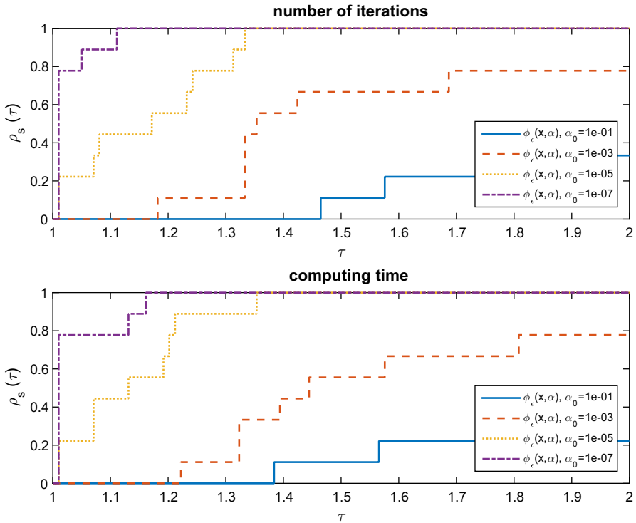
Fig. 4 Performance profile of \phi_\epsilon(x, \alpha) when \alpha_0 = 1e - 1, 1e - 3, 1e - 5 and 1e - 7
